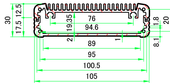
A-A (1:2)
